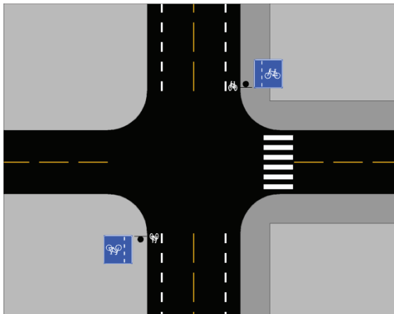
Figur 4.2: Skilting og oppmerking av sykkelfelt i høyreregulert X-kryss
