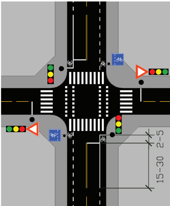
Figur 4.7: Tilbaketrukket stopplinjje for motorvogn i signalregulert kryss (mål i m)
