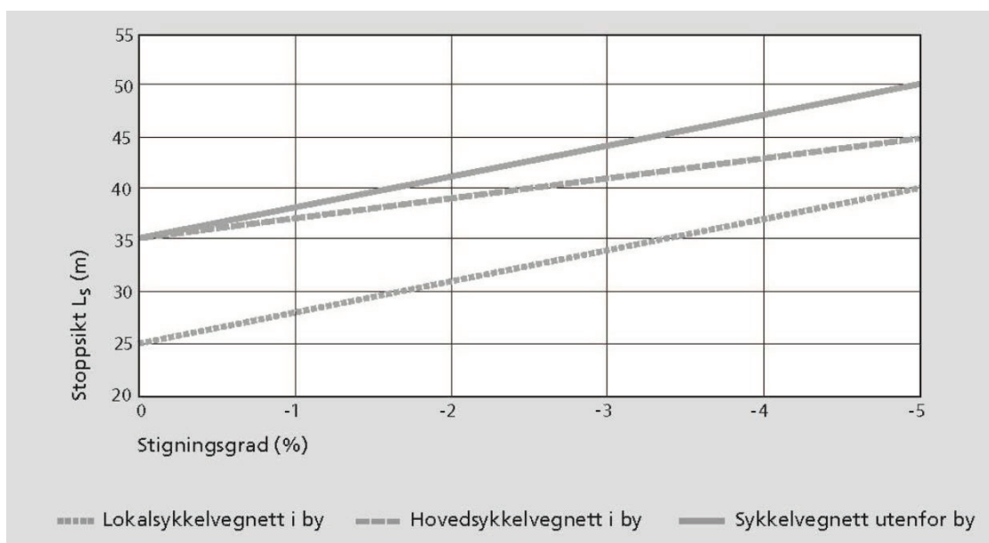
Figur 4.23: Stopsikt ( L_s ) for syklende avhengig av type nett, omgivelser og stigningsgrad
